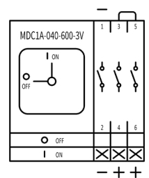
MDC1A 040-600-3 V IEC
