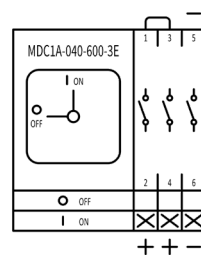
MDC1A 040-600-3 E IEC
