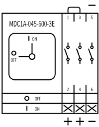
MDC1A 045-600-3 E IEC
