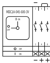
MDC1A 045-600-3 V IEC
