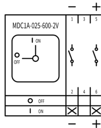
MDC1A 025-600-2 V IEC
